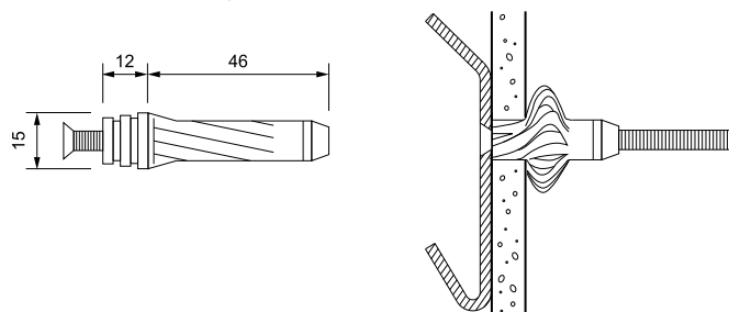
Однослойный гипсокартон
